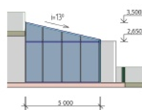
Фасад в осях 4-2
