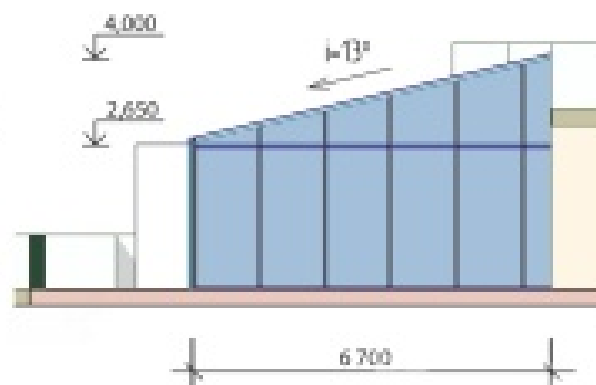
Фасад в осях 2-4
