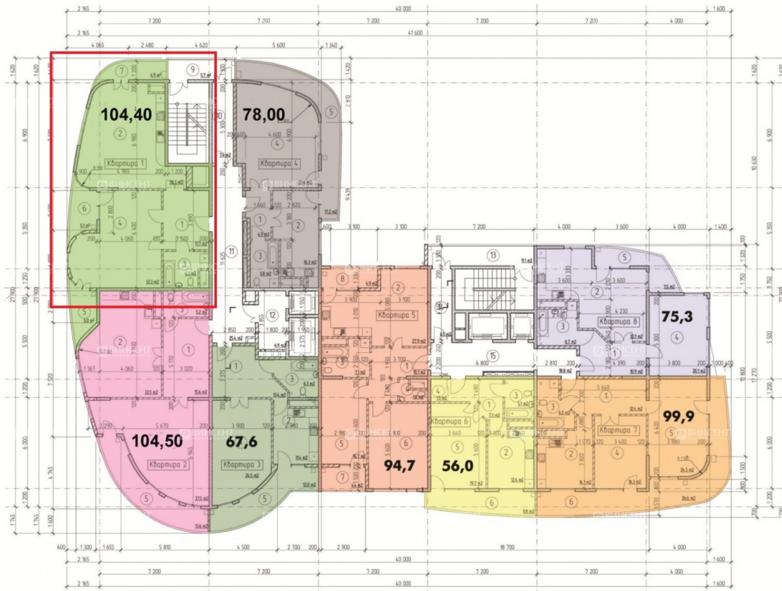
План типового этажа (4-13)
