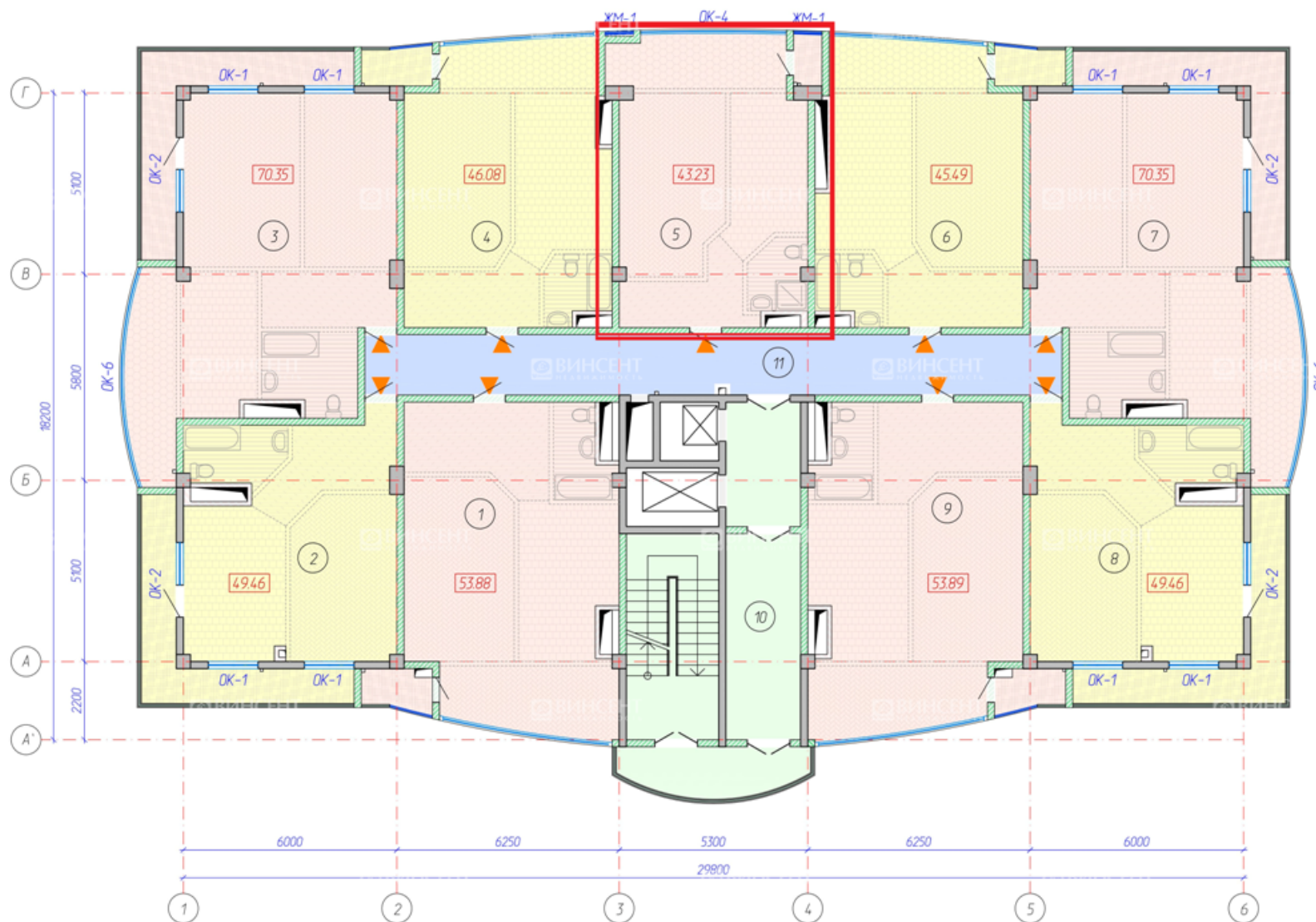
План этажа на отм +3,300, +23,100...+32,700 М 1:100
